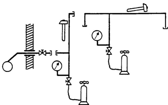
Εικόνα 1 Δοκιμή αντοχής
