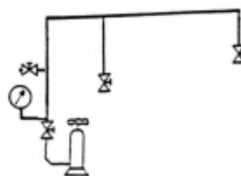
Εικόνα 2 Δοκιμή στεγανότητας
